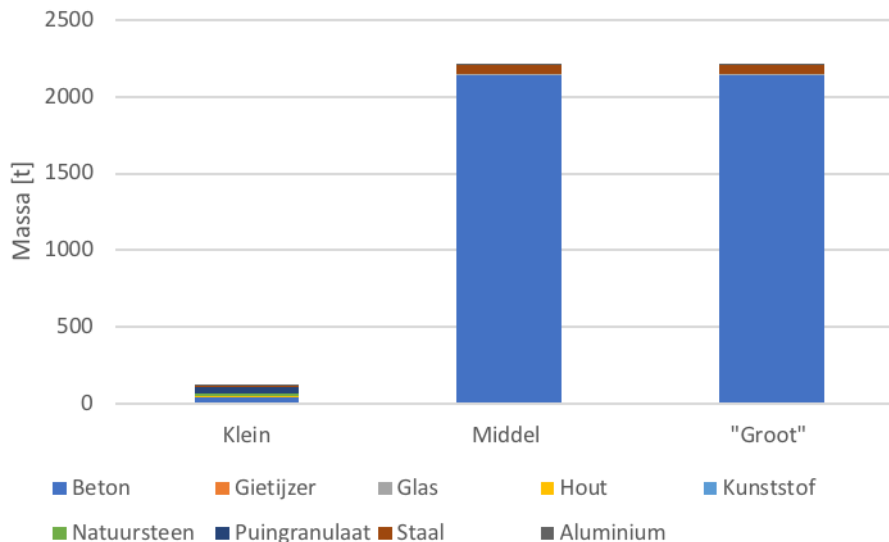
AFBEELDING 3.5 MATERIALISATIE REFERENTIE POLDERGEMALEN
